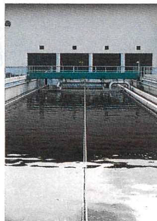
Nachklärbecken
