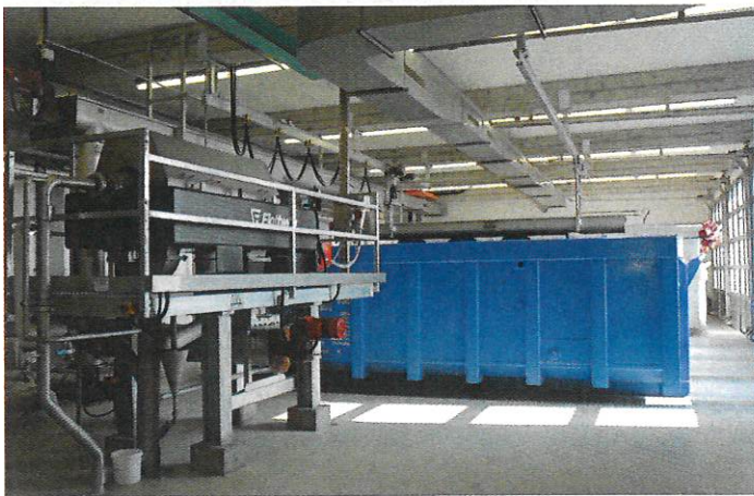
Faulschlammentwässerung
