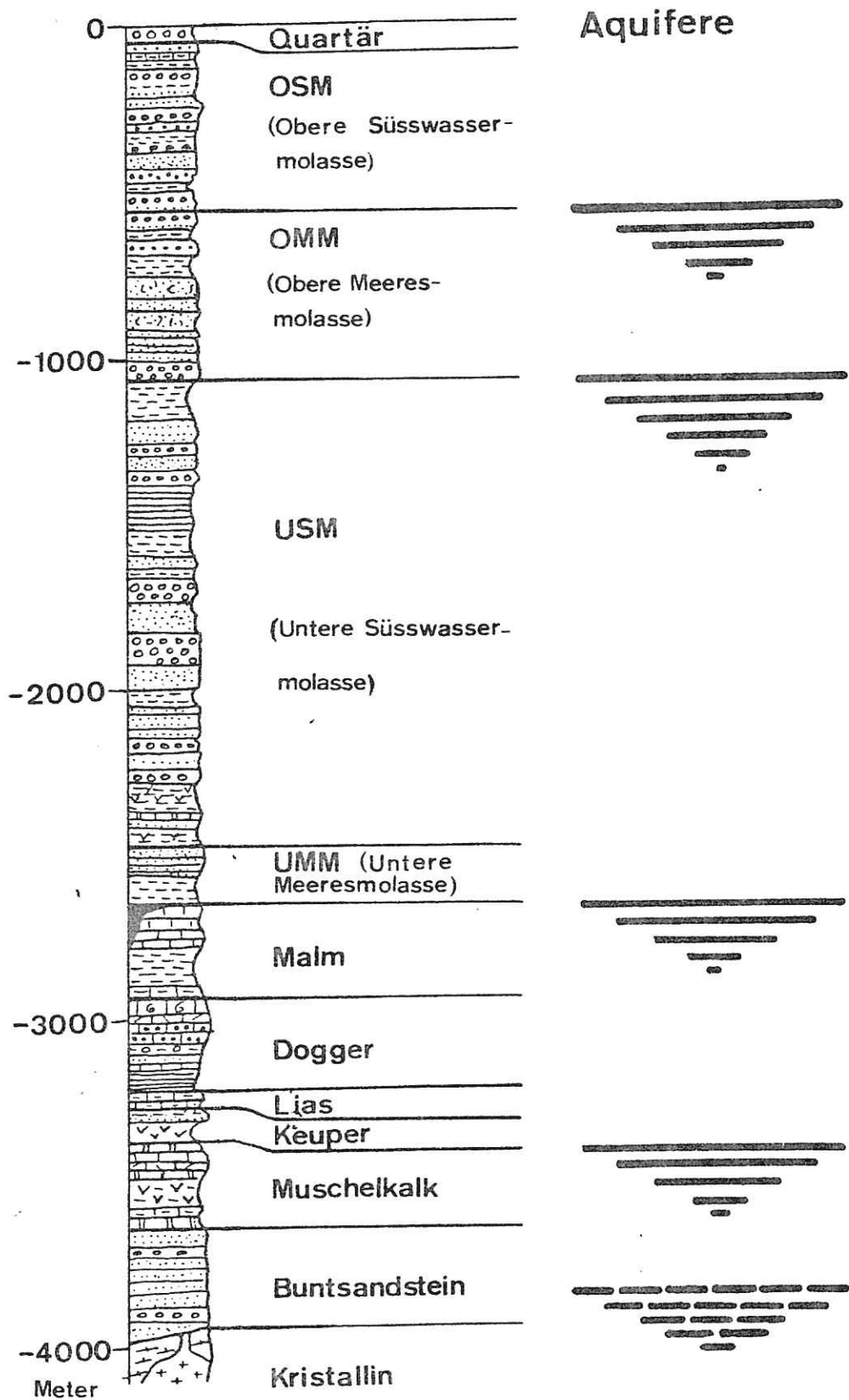
Schematisches stratigraphisches Profil durch das Mittelland
