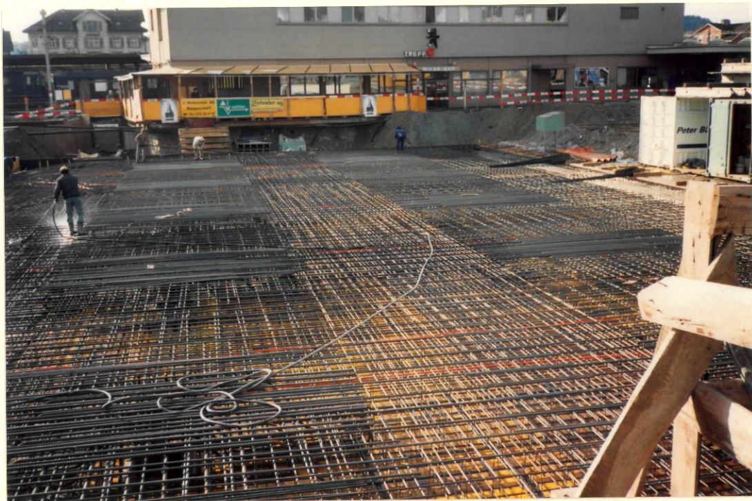
Schalung D e c k e für 1.Untergeschoss 2. Teil 19. November 1991
