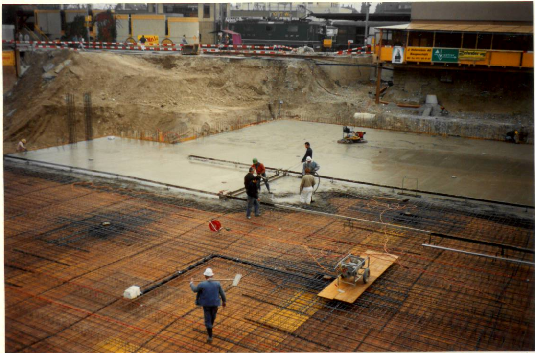
D e c k e 2. Untergeschoss 2. Teil 28. Oktober 1991
