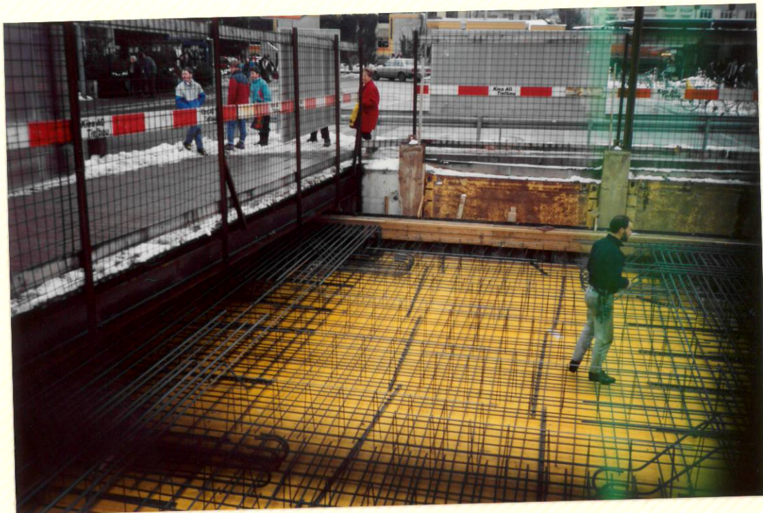
Schalung D e c k e für Durchgang zum Migros 19. Dezember 1990
