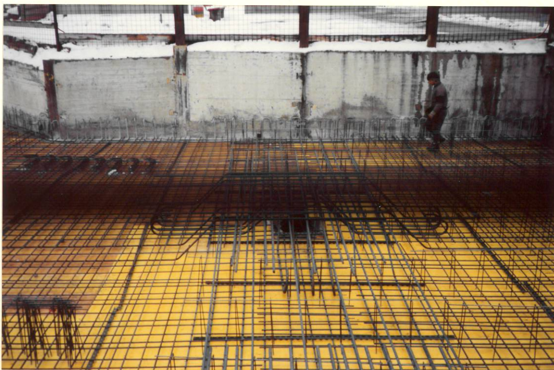
Schalung D e c k e für 1. Untergeschoss 2. Teil 19. Dezember 1990
