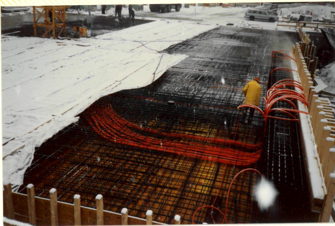
Schalung D e c k e für 1. Untergeschoss 2. Teil 12. Dezember 1990
