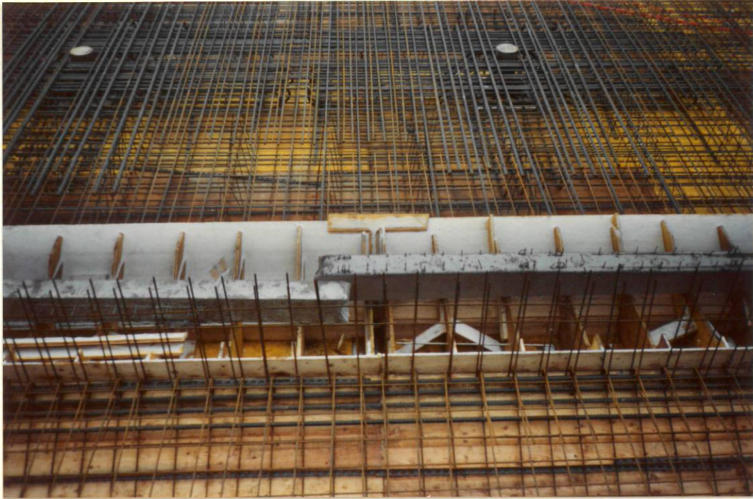
D e c k e für 1. Untergeschoss 2. Teil 3. Dezember 1990
