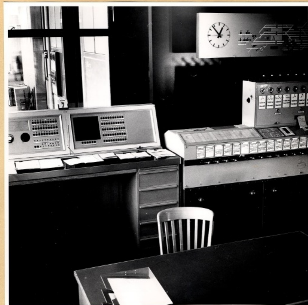
No. 124: Fahrdienstbüro, links Fernmeldepult
